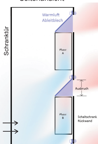
Schaltschrank Seitenansicht
