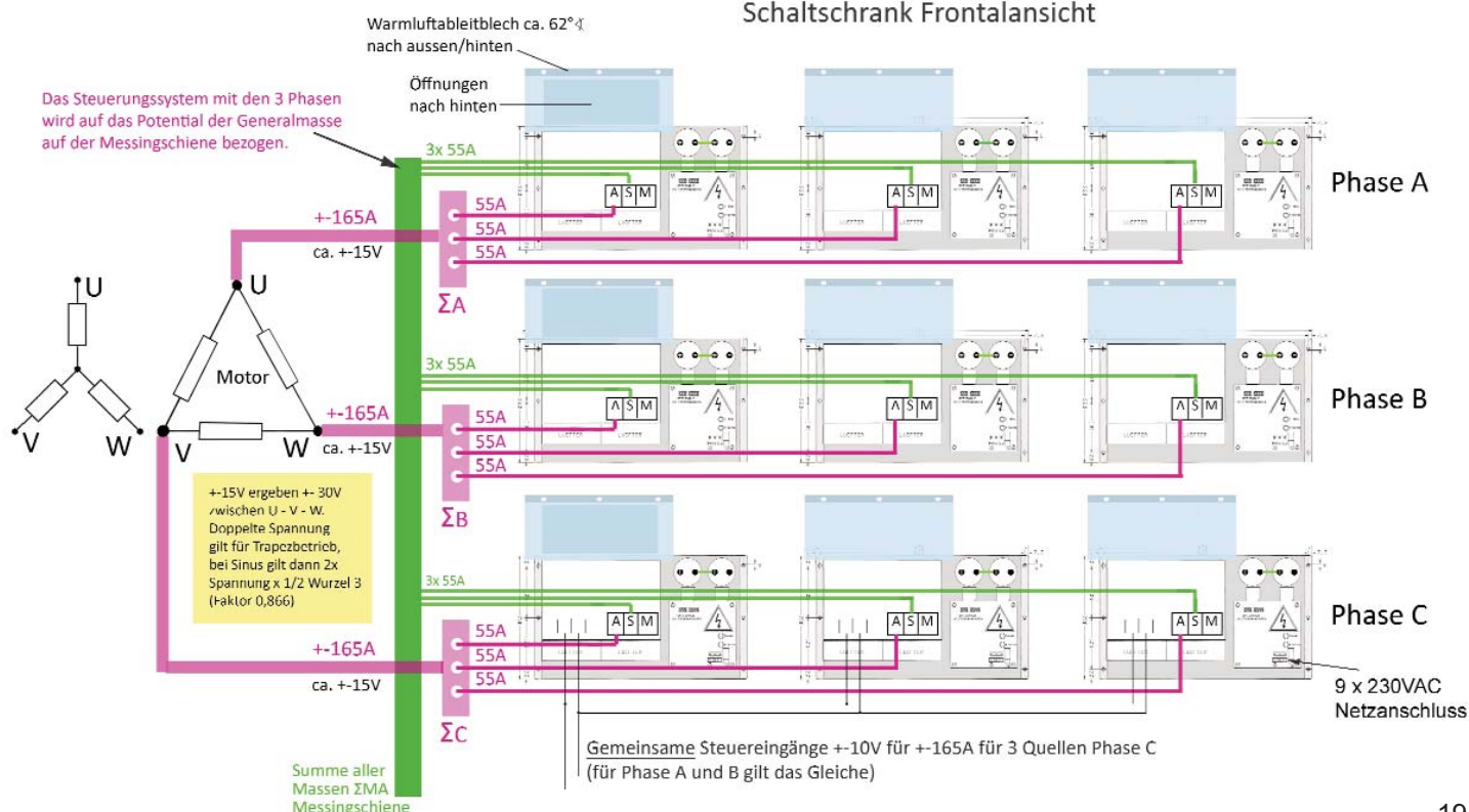
Schaltschrank Frontalansicht
